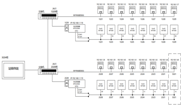
组网拓扑图
